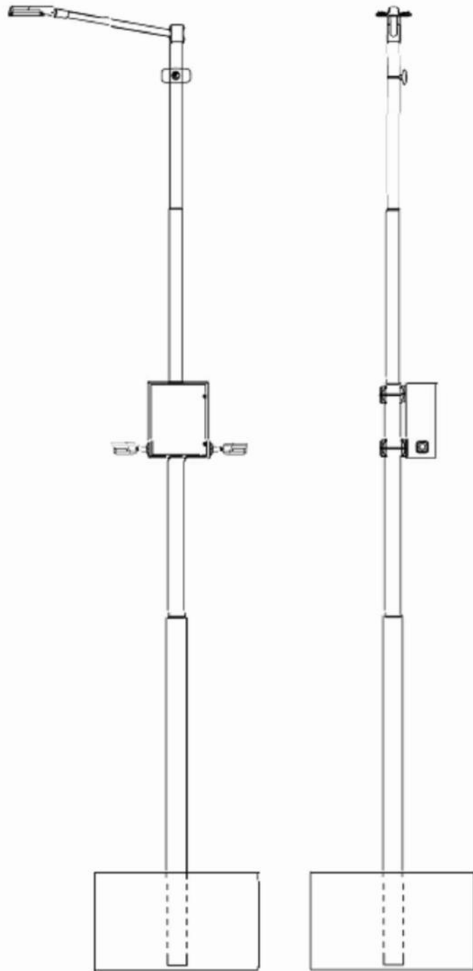
Simulazione Installazione Apparati
