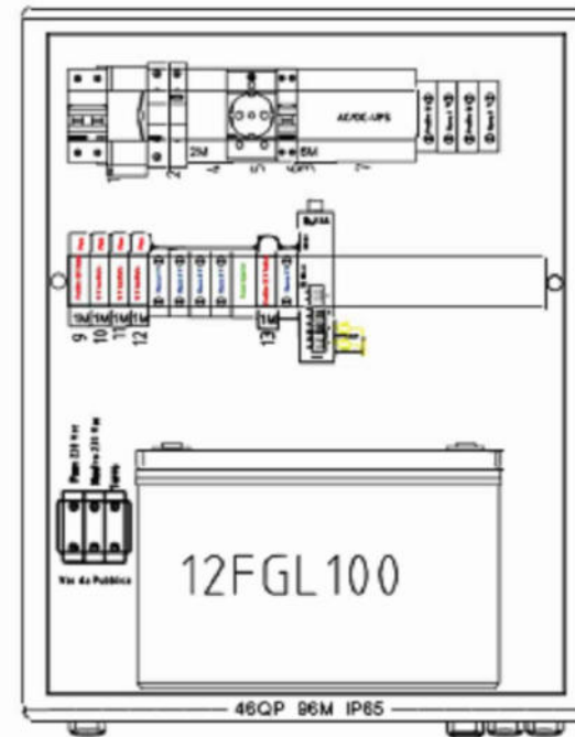
Simulazione Interno Armadio di Campo
